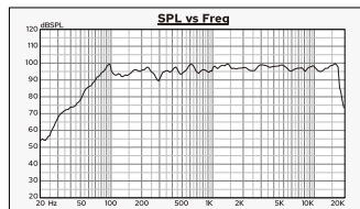
PS-100频响曲线
