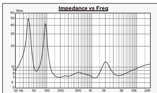
PS-100阻抗曲线
