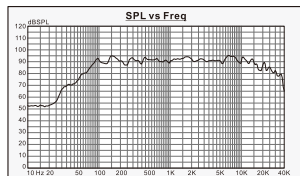
PS-60频响曲线
