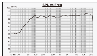
PS-150频响曲线
