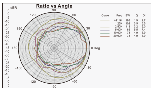
PS-60指向性(极坐标)
