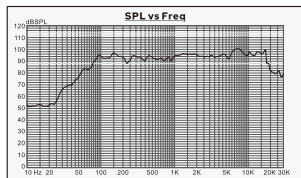
PS-80频响曲线
