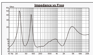
PS-120阻抗曲线
