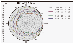
PS-80指向性(极坐标)
