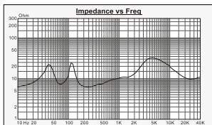
PS-60阻抗曲线
