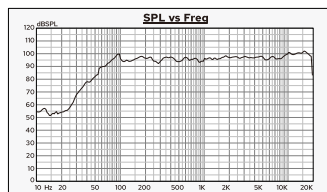
PS-120频响曲线
