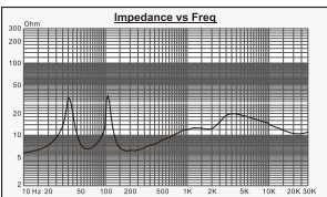
PS-80阻抗曲线
