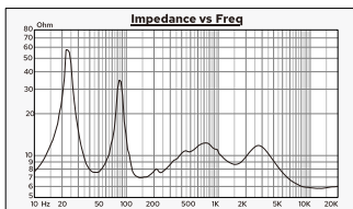
PS-150阻抗曲线
